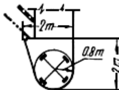
Мельница молотковая с тангенциальным подводом воздуха
