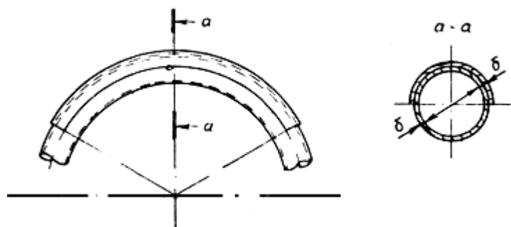
Рис. 1. Расположение противоизносной накладки
