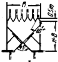
Коробка воздухораспределительная для двух вентиляторов с переключающими шиберами
