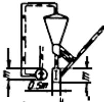
Мельница аэробильная с сепаратором и вентилятором
