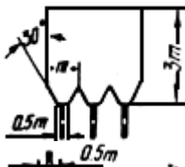
Бункеры пылевидного топлива (длина бункера определяется числом пылепитателей)
